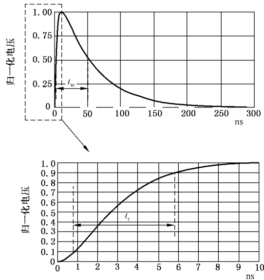
图 3 输出到 50 \Omega 负载的单个脉冲的理想波形 ( t_r = 5 \text{ ns} , t_w = 50 \text{ ns} )
